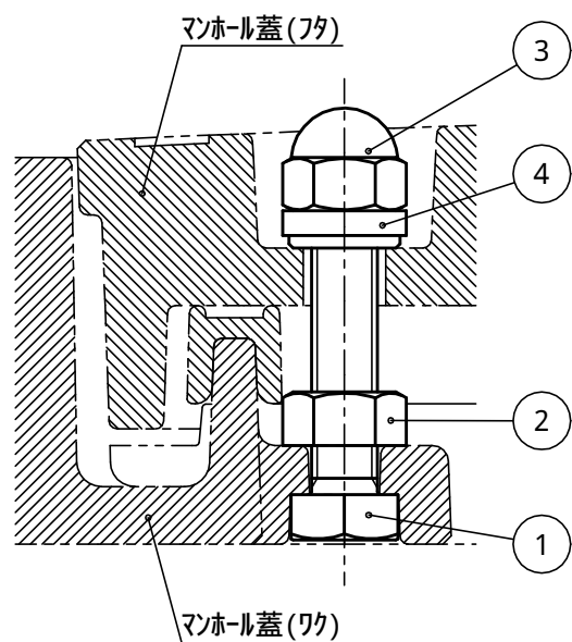
P部拡大図 (1/1)
